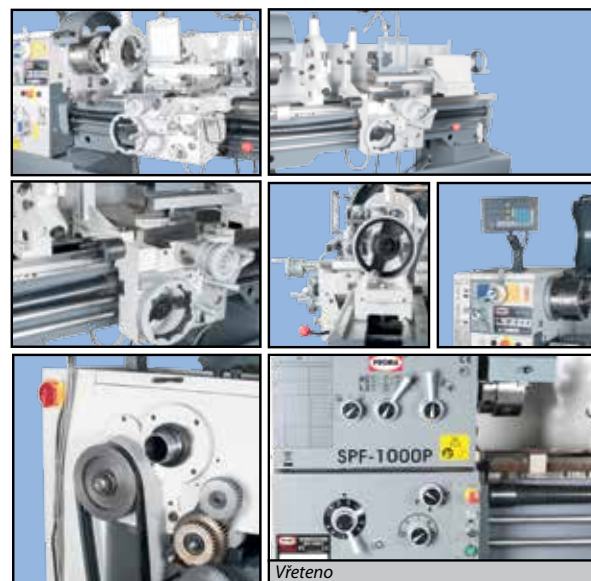
Vřeteno
